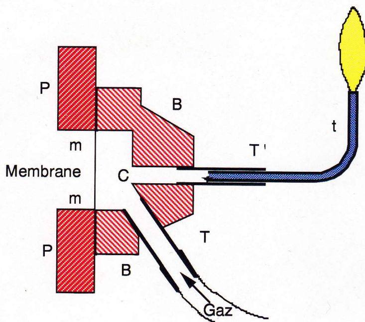
Capsule manométrique de KOENIG
